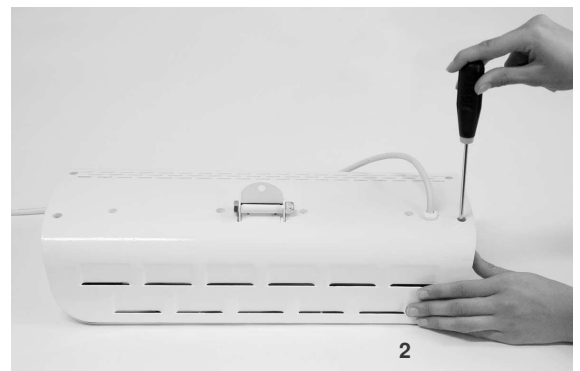
2. ОТКРУТИТЕ 4 ВИНТА С ОБРАТНОЙ СТОРОНЫ КОРПУСА ОБОРУДОВАНИЯ
