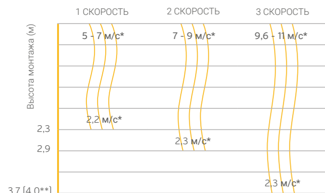
Длина вертикальной струи воздуха (максимальная высота монтажа)
