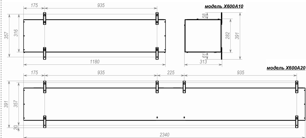
Рис. №1 Габаритные и установочные размеры завес X600A10 и X600A20
