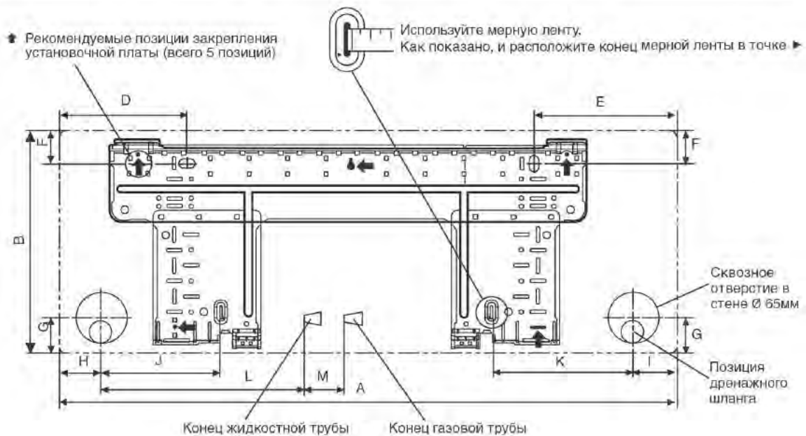
МОНТАЖНАЯ ПЛИТА 20/25/35
