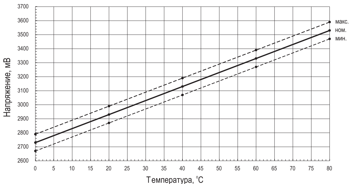
Рис.3 Напряжение на датчике в зависимости от температуры
